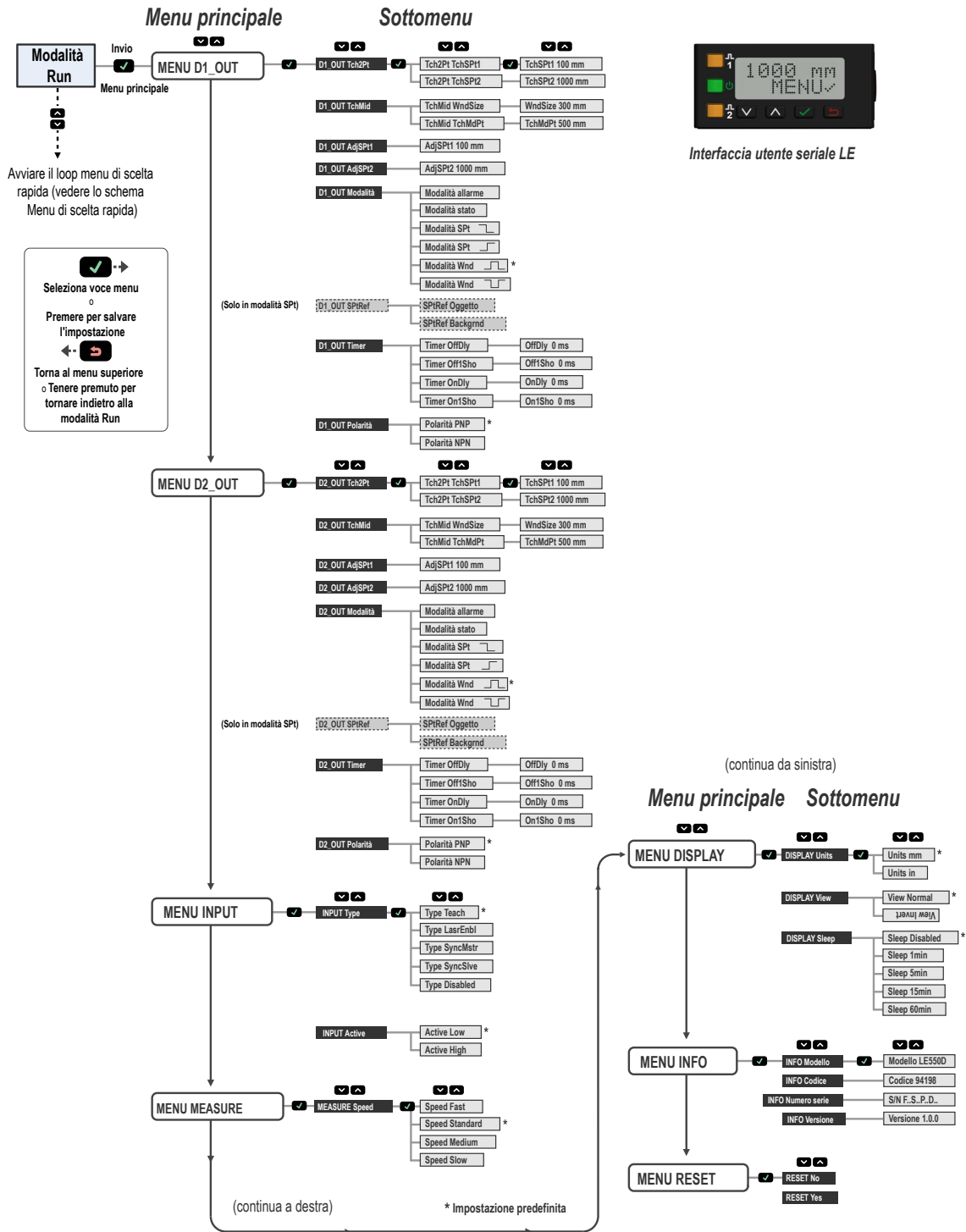
Figura 13. Menu sensore LE550 - Mappa (modelli digitali doppi)
