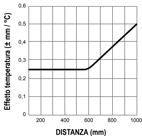
Figura 17. Effetti della temperatura
