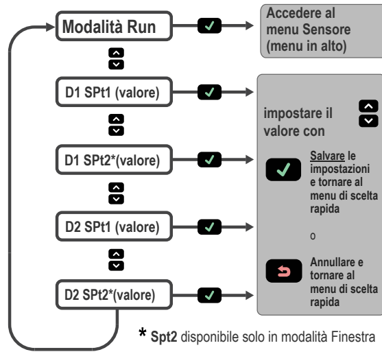
Figura 12. Mappa menu di scelta rapida (Modalità campo)
