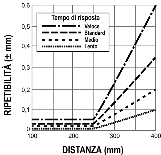
Figura 14. Ripetibilità (riflettanza dal 90% al 6%)
