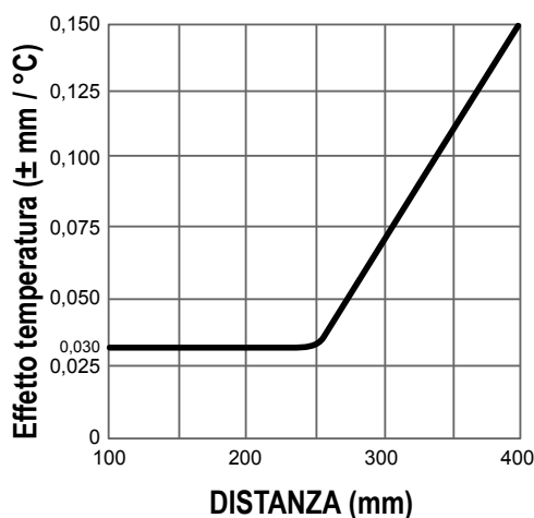
Figura 16. Effetti della temperatura
