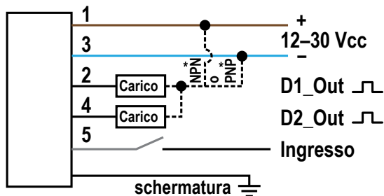
Figura 9. Modelli con due uscite digitali
