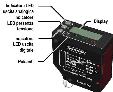
Figura 1. Caratteristiche del sensore digitale doppio LE
