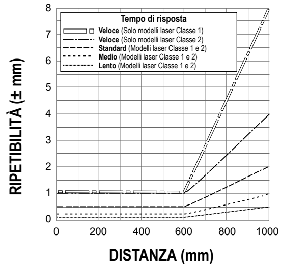
Figura 15. Ripetibilità (riflettanza dal 90% al 6%)
